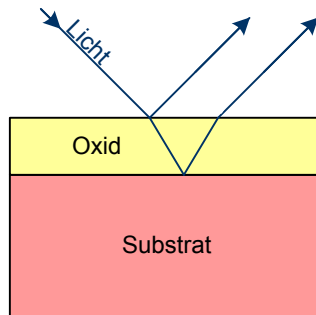
Abb. 1.2: Ellipsometrie
